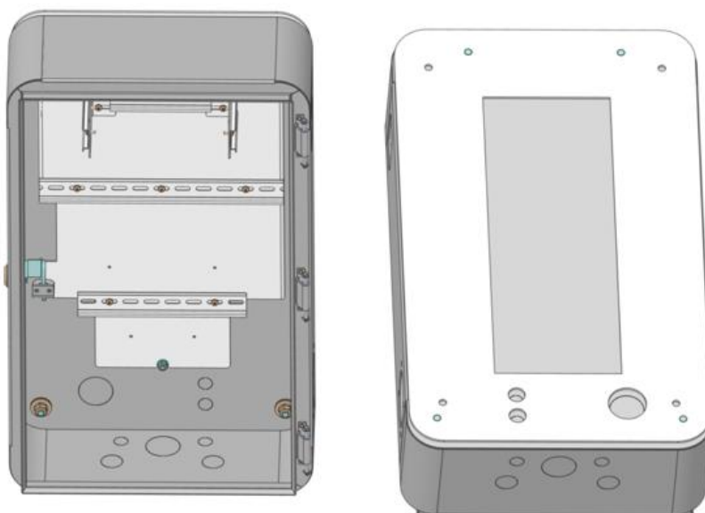
Před-vyražené díry pro kabelové vývodky na přívodní silový a komunikační kabel
