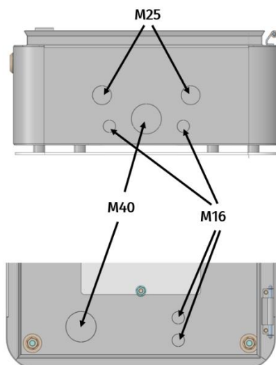
Před-vyražené díry pro kabelové vývodky na přívodní silový a komunikační kabel
